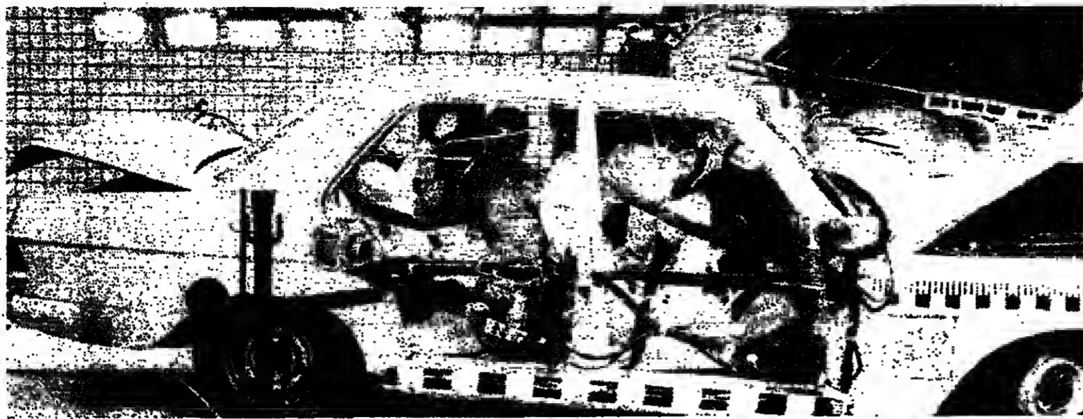
Beim Aufprall wurden der Gepäckträger abgerissen und die nicht angeschalteten Dummies gegen das Armaturenbrett geschleudert.
